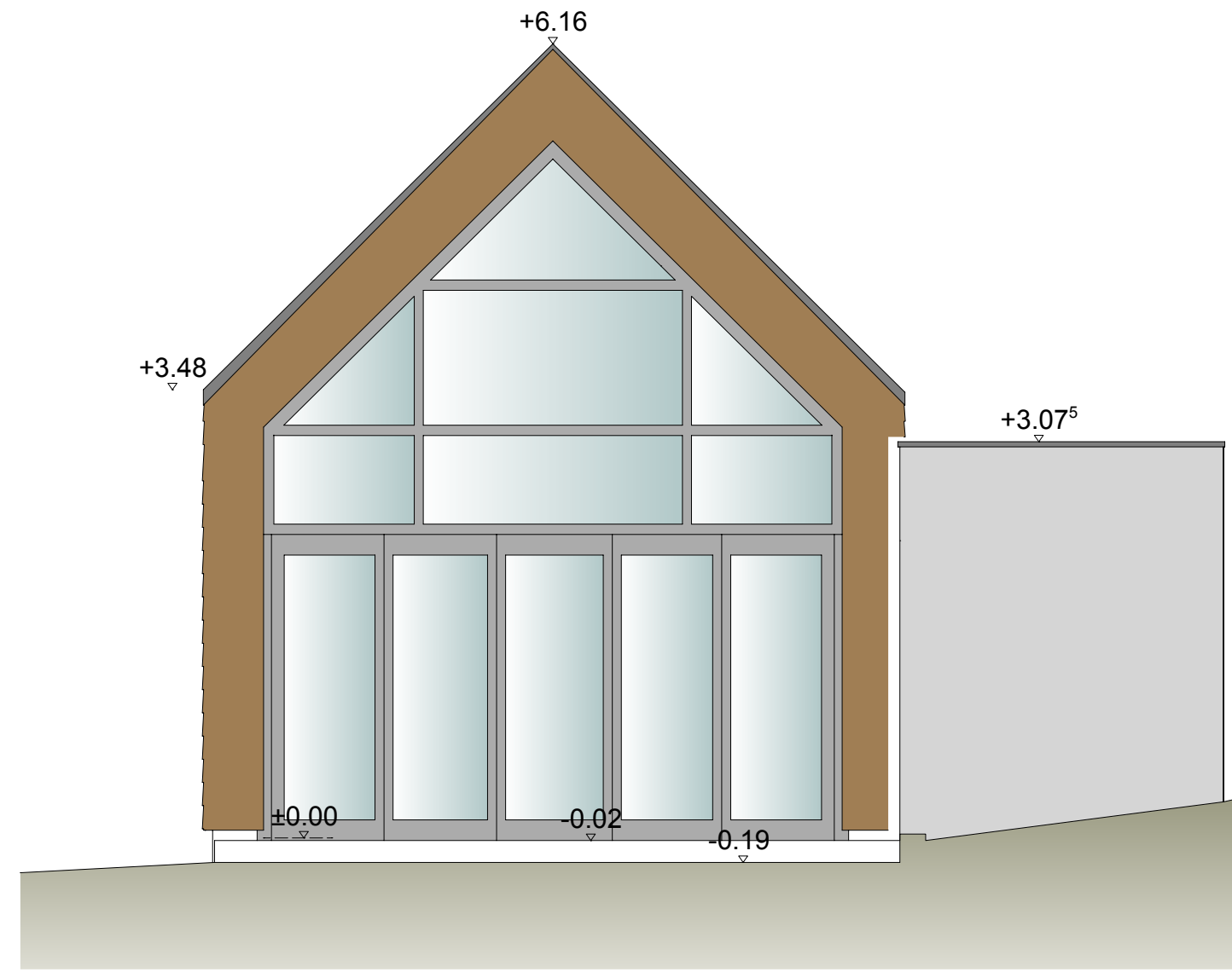
Ansicht Osten
