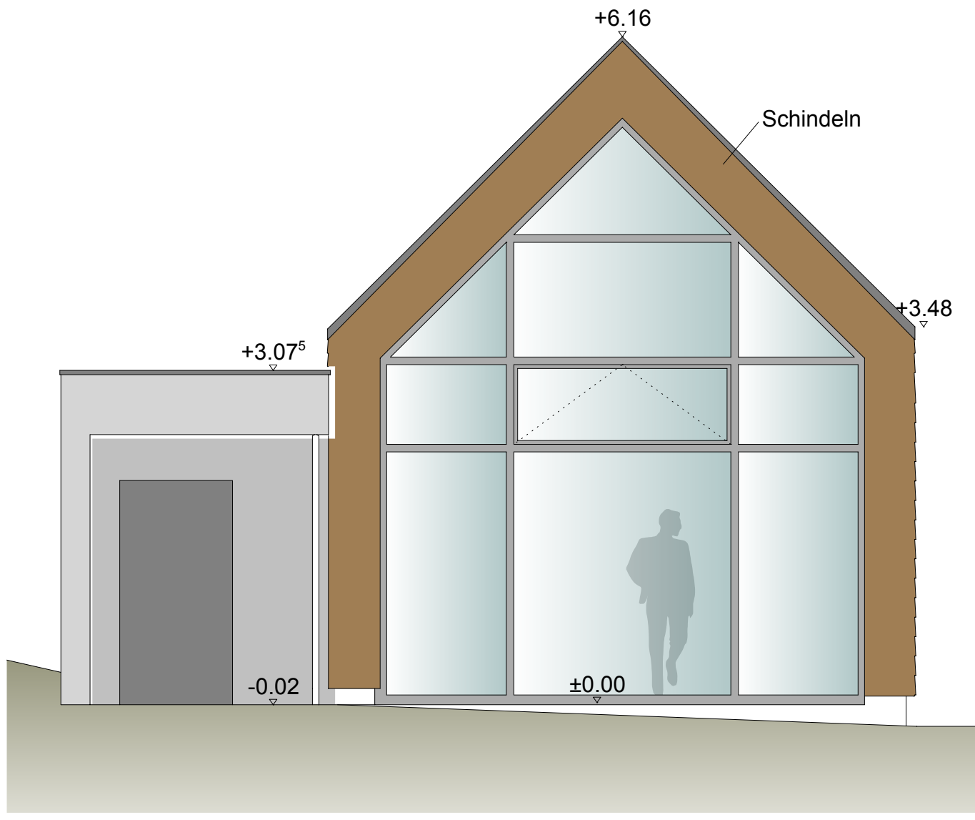
Ansicht Westen
